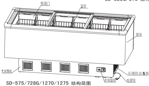
SD-575/728G/1270/1275 结构简图
