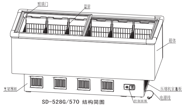
SD-528G/570 结构简图
